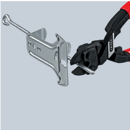
mit Greiffläche unter dem Gelenk zum Greifen und Ziehen von Drähten ab \varnothing 1,0 mm
