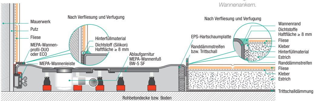
Abbildung Montage mit Quick-Set Typ SF
