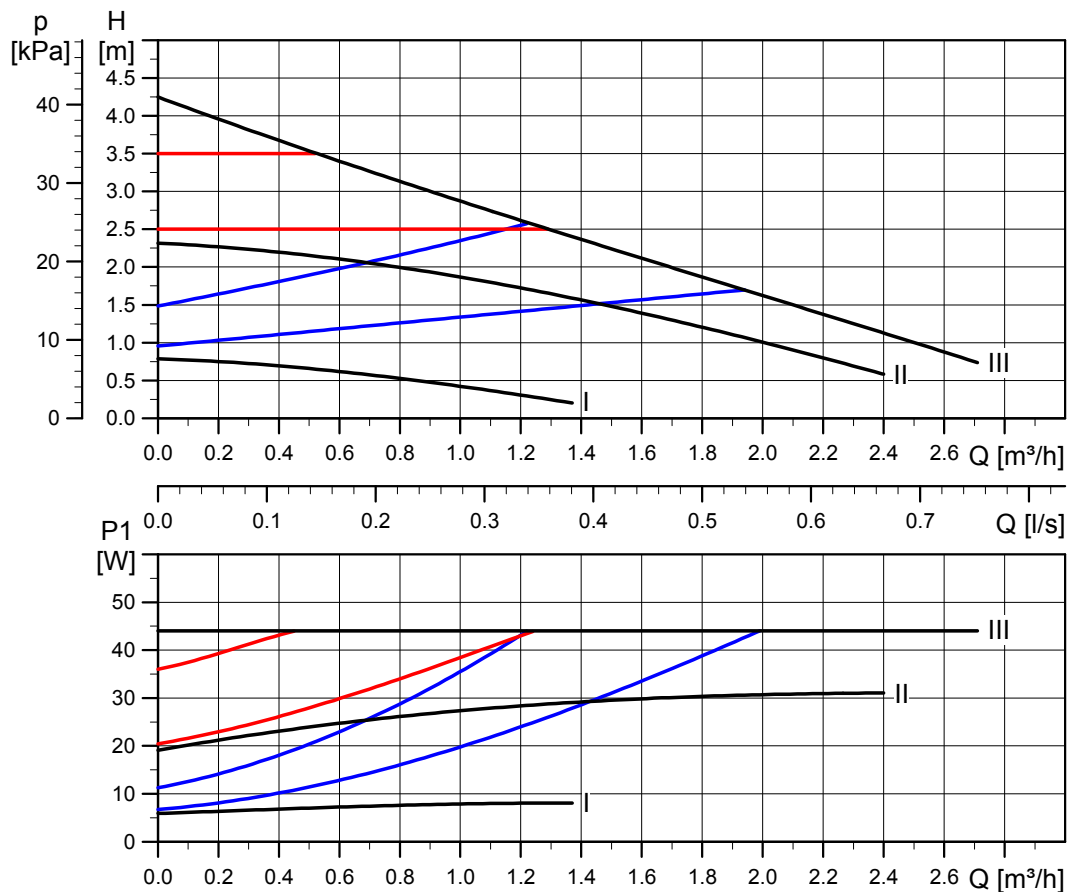
Abb. 19 Kennlinien, ALPHA2 L 20-45
