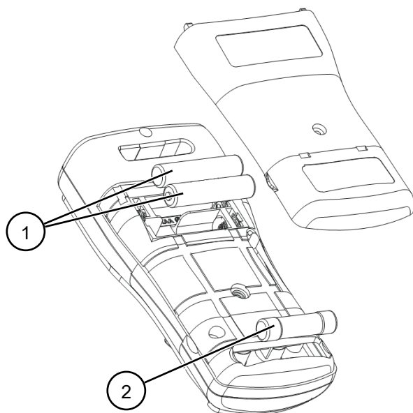
Illustration 16: Remplacement des piles (exemplaire)
