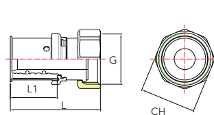
ÜBERGANGSPRESSVERSCHRAUBUNG FLACHDICHTEND / RACCORD À SERTIR ET ÉCROU TOURNANT JOINT PLAT
