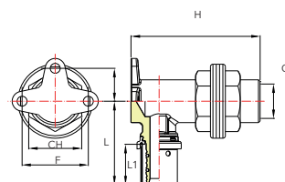
WANDDURCHFÜHRUNG AG/IG MIT VERDREHSCHUTZ
