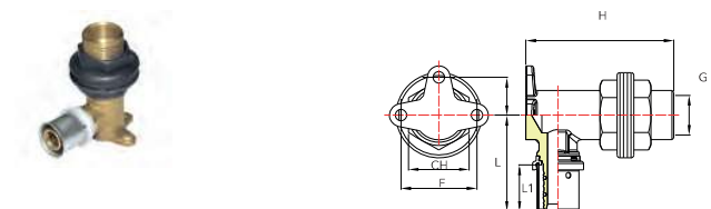
WANDDURCHFÜHRUNG AG/IG MIT VERDREHSCHUTZ
