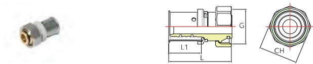
ANSCHLUSSPRESSVERSCHAUBUNG MIT EUROKONUS / RACCORD À SERTIR ET ÉCROU TOURNANT EUROCÔNE
