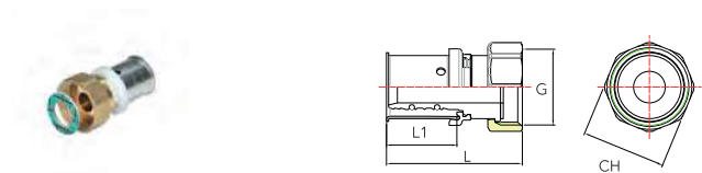
ÜBERGANGSPRESSVERSCHAUBUNG FLACHDICHTEND / RACCORD À SERTIR ET ÉCROU TOURNANT JOINT PLAT
