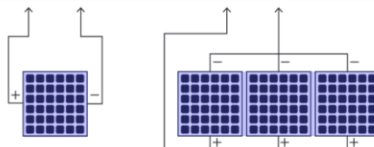
Parallelschaltung von x Photovoltaikmodulen als Referenz
