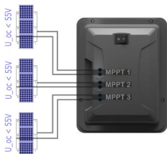
Anschluss eines Beispielsystems (3x 300W 60 Zellen Modul pro MPP Tracker, gesamt 2700Wp)
