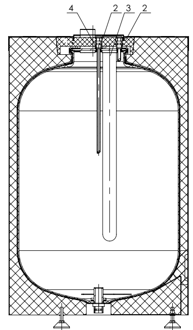
ABSCHNITT C-C
