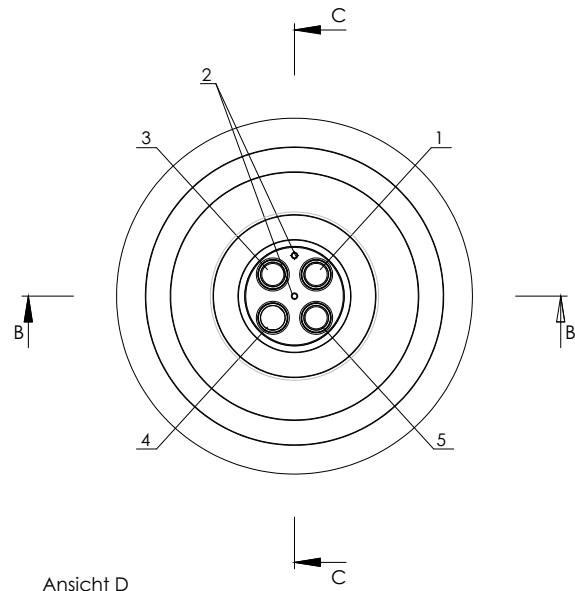
Ansicht D
