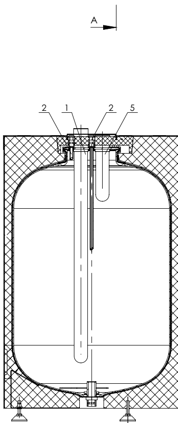
ABSCHNITT A-A
