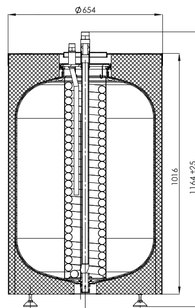
ABSCHNITT A-A
