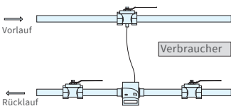
Asymmetrischer Fühlereinbau bei Celsius C5 mit Temperaturenhlertyp TS-45-5 im DFS integriert
