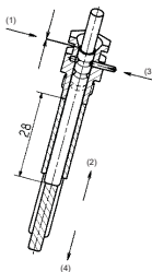
Esempio di montaggio per adattatore in ottone
