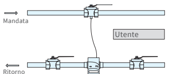
Esempio di montaggio per adattatore in plastica
