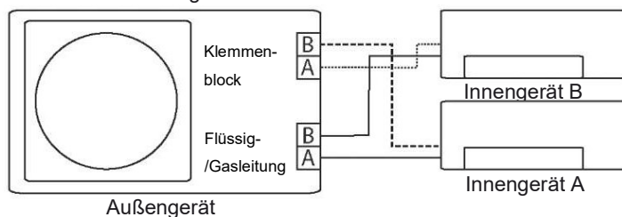
Falsche Verdrahtung
