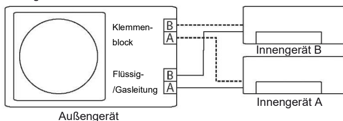
Falsche Verdrahtung
