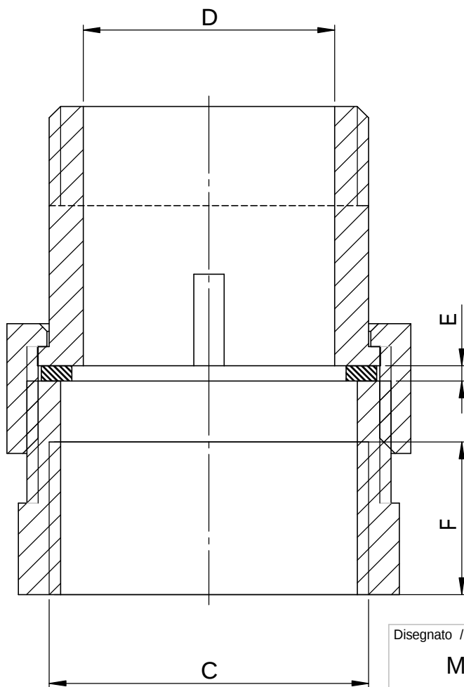
SEZIONE A-A
