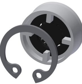
Durchflussmengenregler 9,0 l/min
