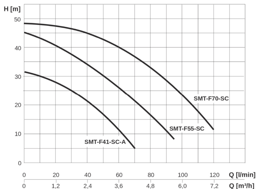
Abb.: Pumpenkennlinie
