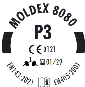
Vorderseite 8080
