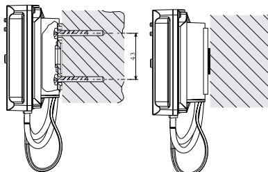
Bague de montage sur une surface plane avec 2 vis (non fournis)
