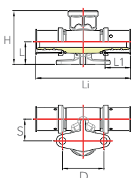
GEGENEINANDER VERDREHTE ENDSTÜCKEN IG /RACCORDS DÉSAXÉS FEMELLE
